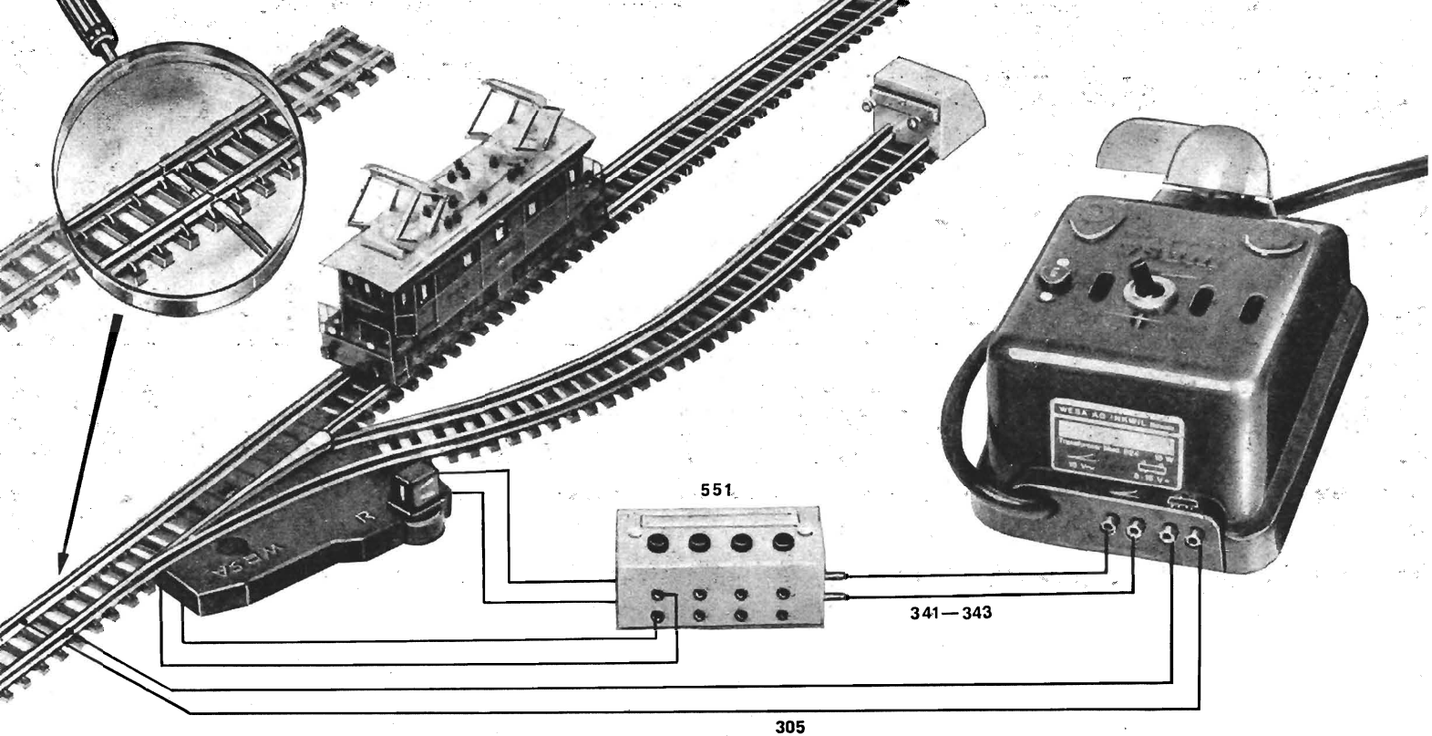
Anschluss-Schema für WESA-Bahnen Le raccordement des Trains-WESA
